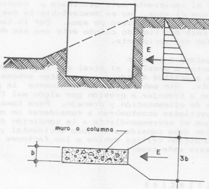
FIGURA C-7.3.1 EMPUJES DE TIERRAS SOBRE MIEMBROS CON LADOS ANGOSTOS
