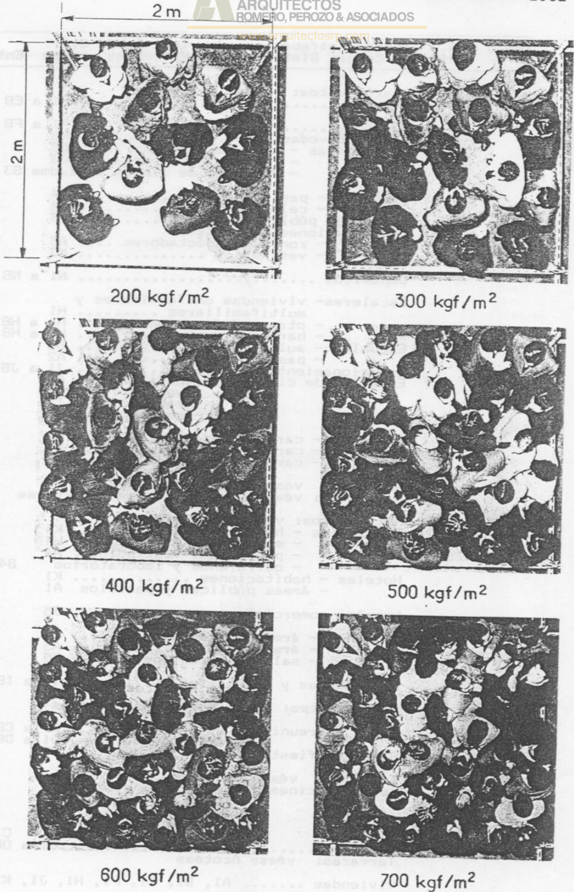
FIGURA C-5.2 ACCIONES VARIABLES DEBIDAS A MUCHEDUMBRES [5.6]
