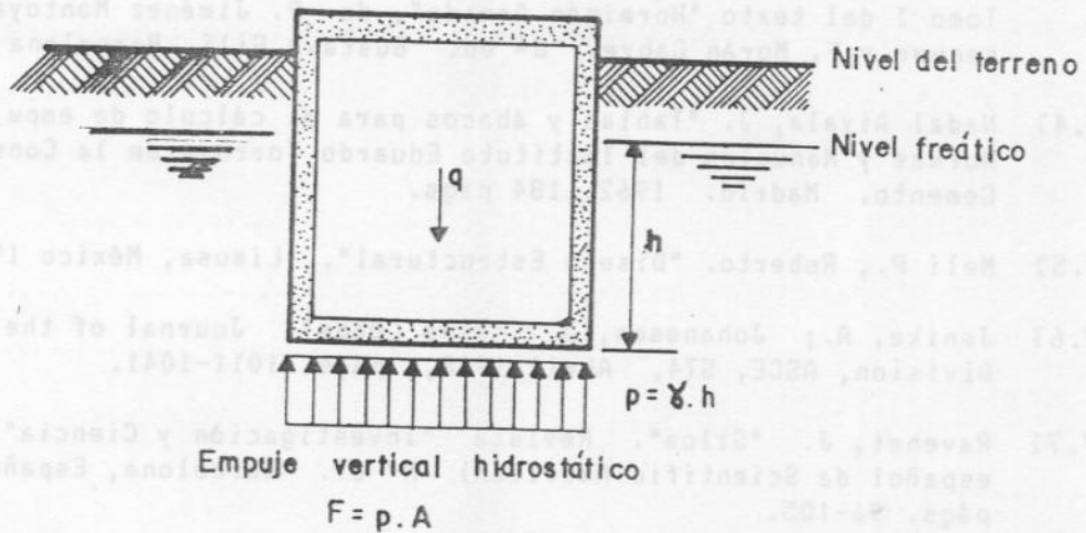
FIGURA C-7.4 SUBPRESION EN UNA ESTRUCTURA ENTERRADA DE PESO TOTAL q Y AREA EN PLANTA A [7.5]
