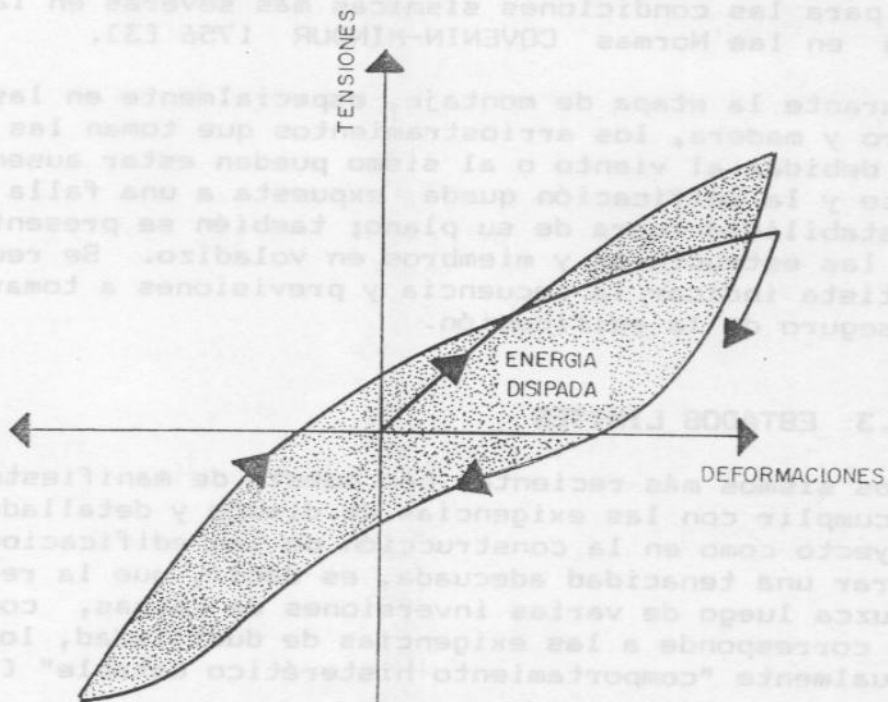
a) COMPORTAMIENTO HISTERETICO ESTABLE
