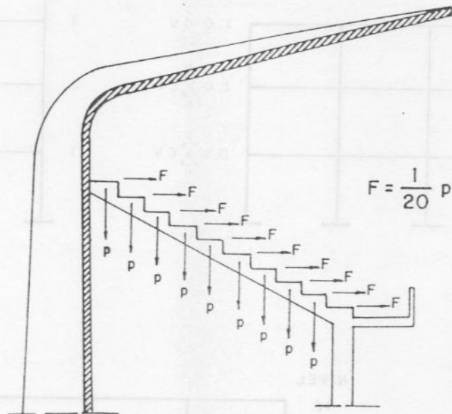
FIGURA C-5.3.1 CARGAS VARIABLES EN TRIBUNAS
